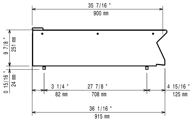
Felülnézet
